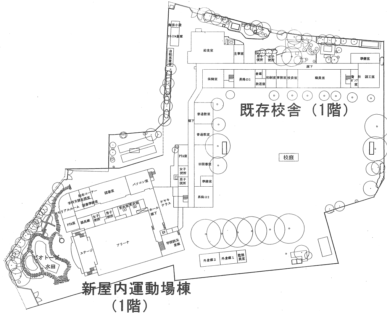
永福小学校 (配置・1階平面図)
