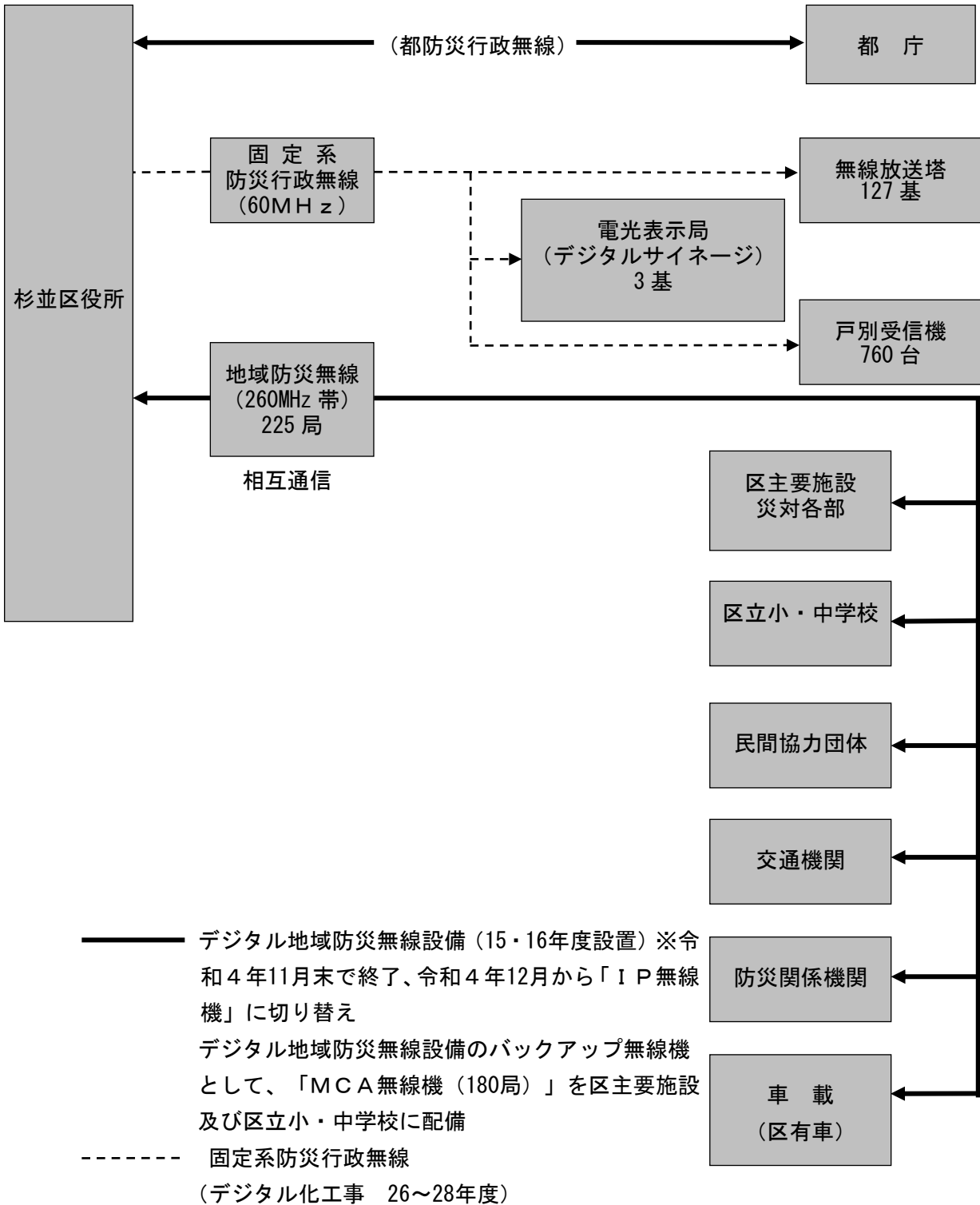
図表：杉並区防災行政無線系統図（令和2年8月現在）
