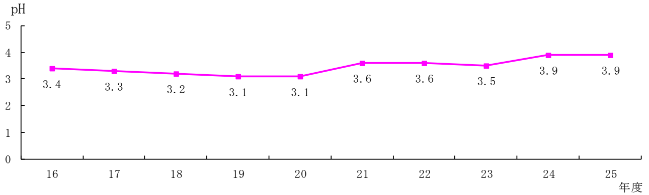
<第3-1-8図> 雨水の pH 最小値の経年変化
