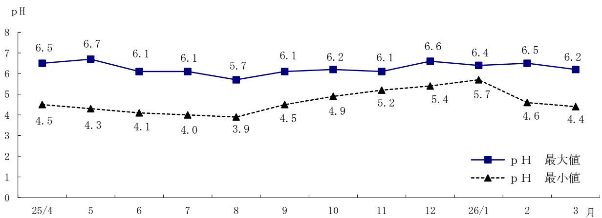
<第3-1-9図> 平成25年度 酸性雨調査結果
