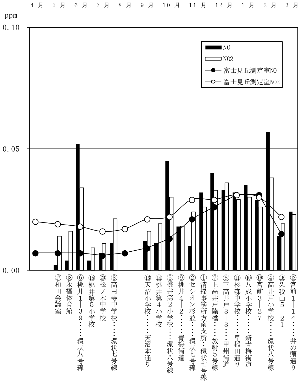
<第3-1-4図> 窒素酸化物連続測定結果（期間平均値：平成25年度）
