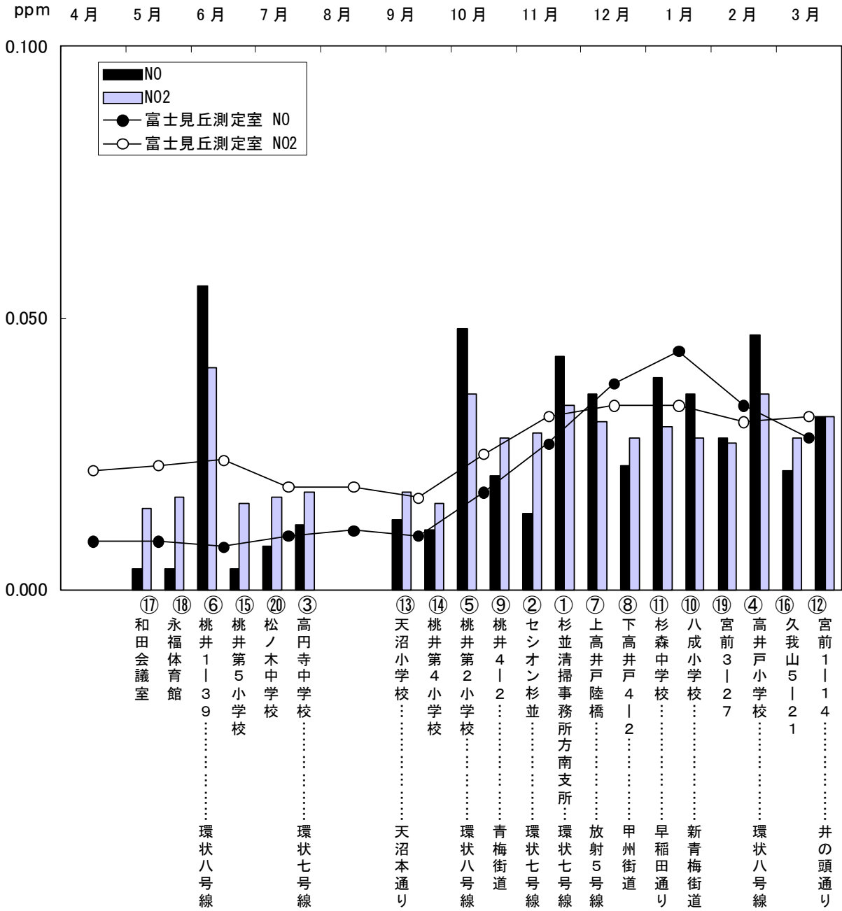
<第3-1-4図> 窒素酸化物連続測定結果（期間平均値）
