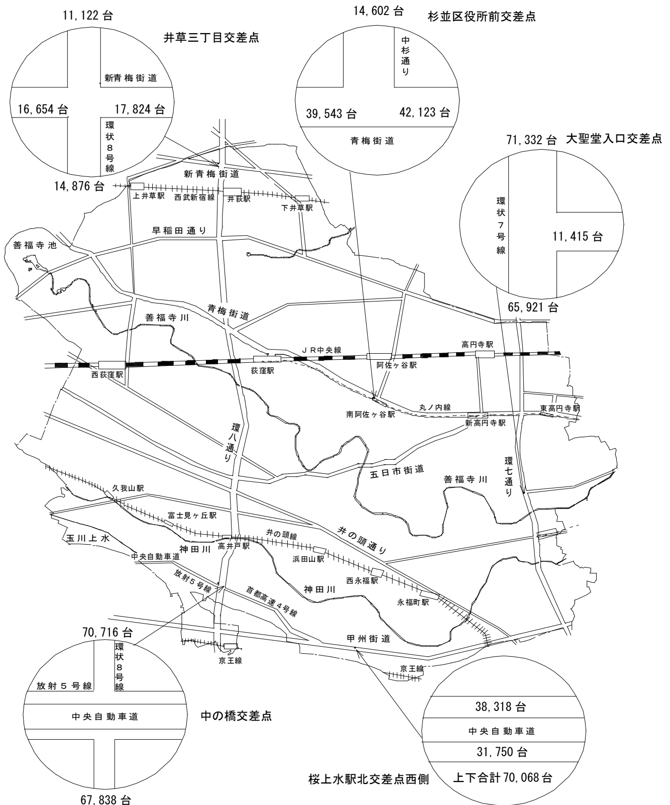
<第3-2-3図> 交通量調査地点と24時間交通量
