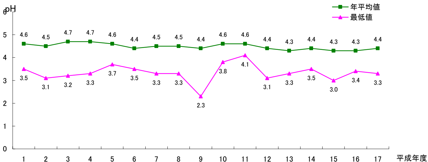
<第1-1-8表> 平成17年度 酸性雨調査結果
