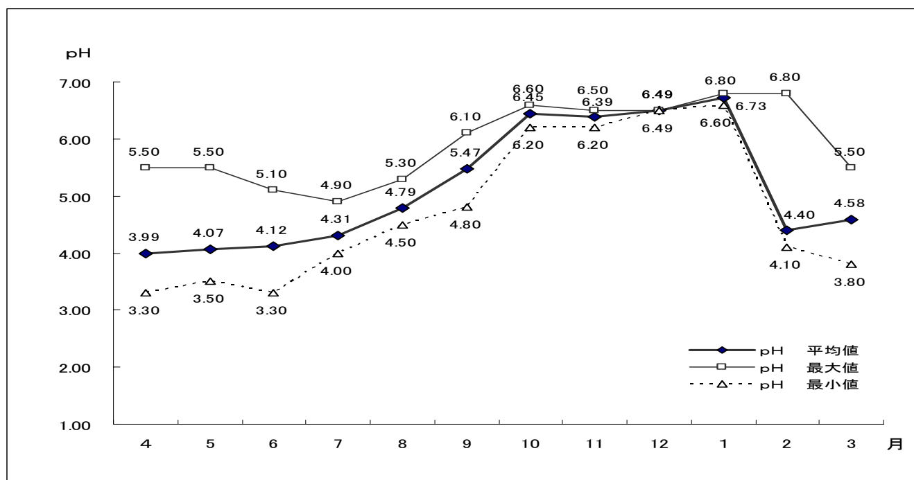
<第1-1-9図> 平成17年度 雨水のpHの月別変化
