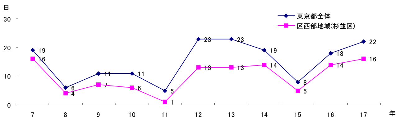
<第1-1-7図> 光化学スモッグ注意報発令回数の経年変化
