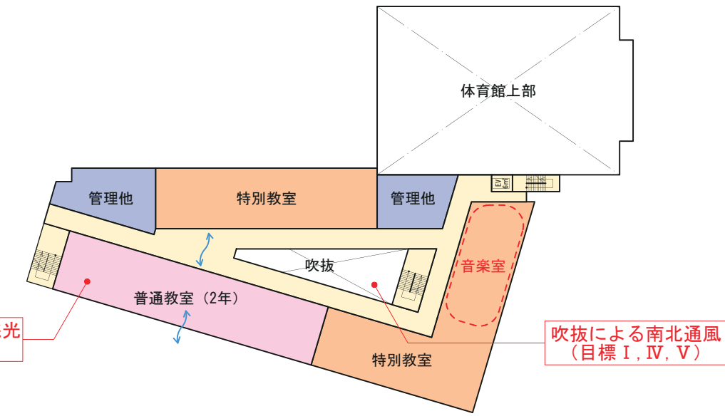
3階平面図
