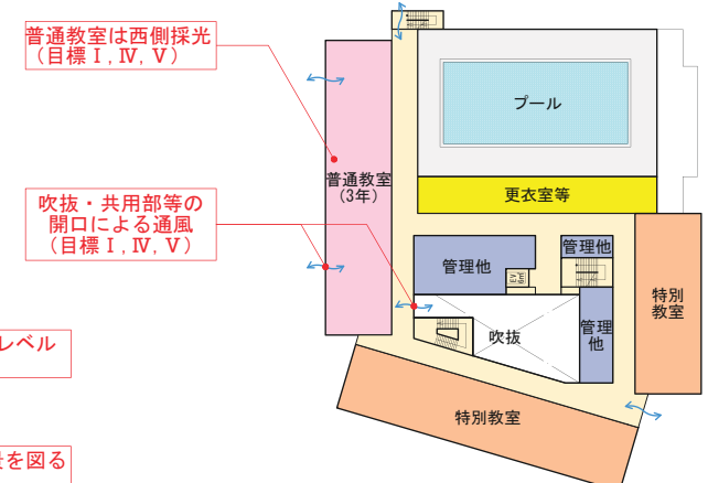
4階平面図
