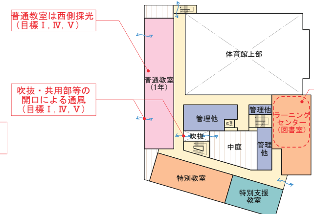
2階平面図
