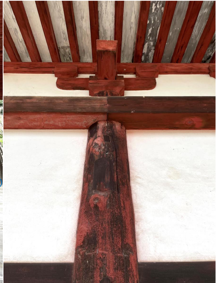
柱頭見上げ写真
