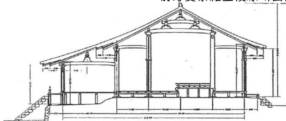
前身曼荼羅堂復原断面図(孫庇付)
