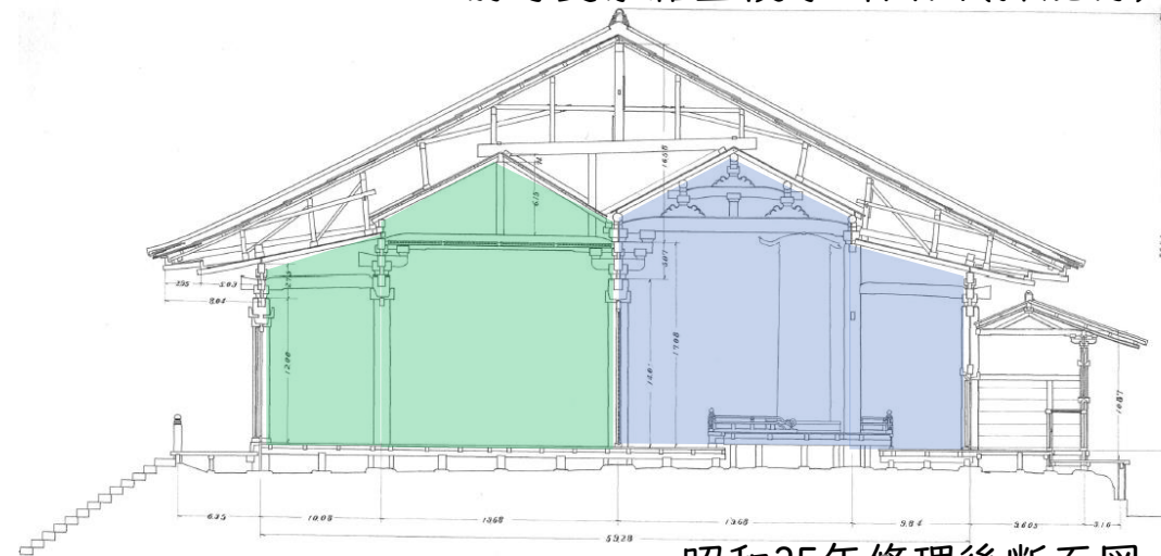
昭和35年修理後断面図
