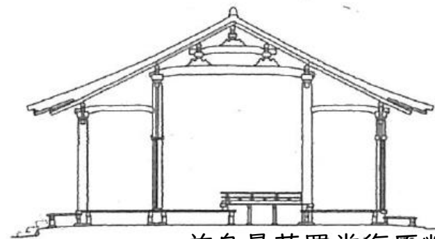
前身曼荼羅堂復原断面図
