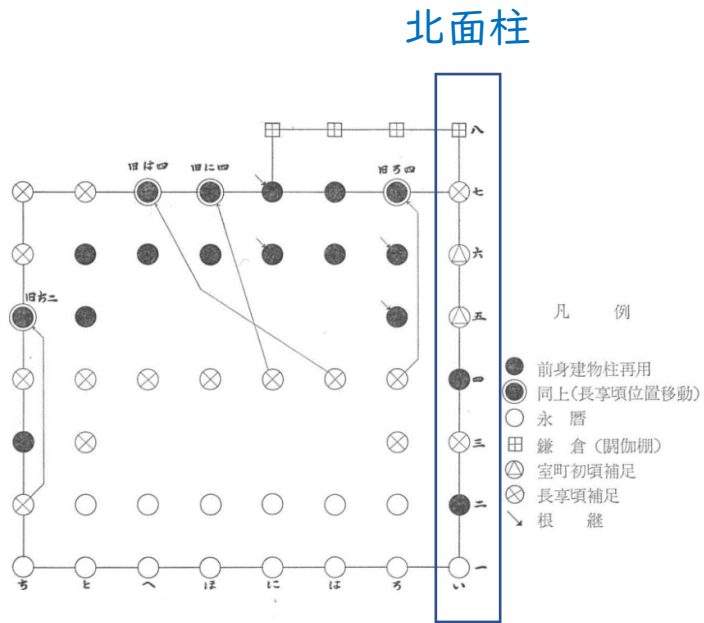
柱分類図
