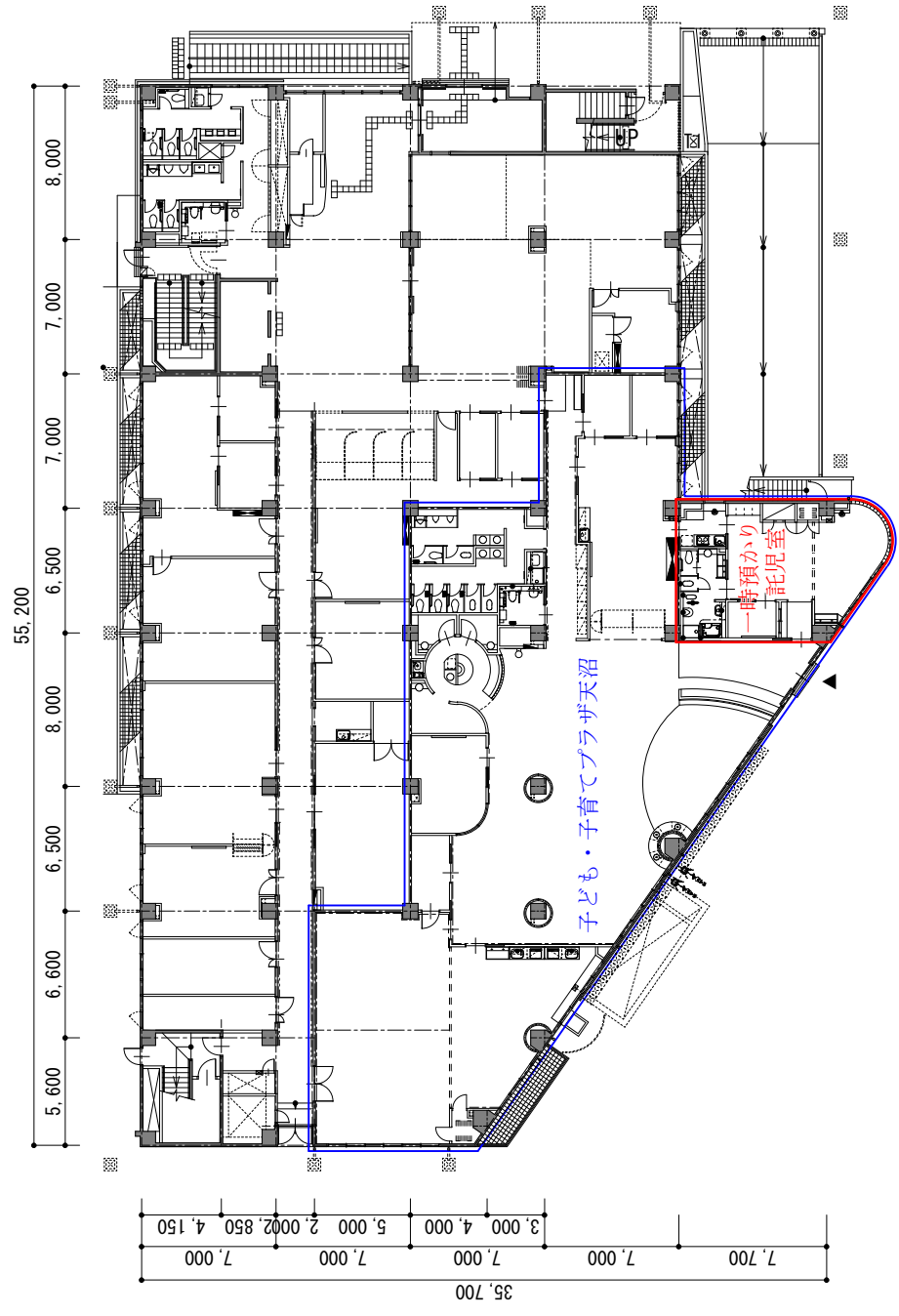
杉並区立子ども・子育てプラザ天沼 1階平面図
