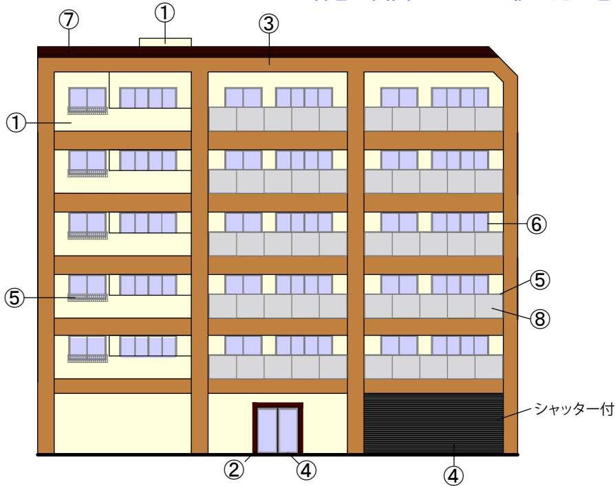
南立面図 1/100
