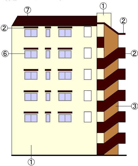
東立面図 1/100
